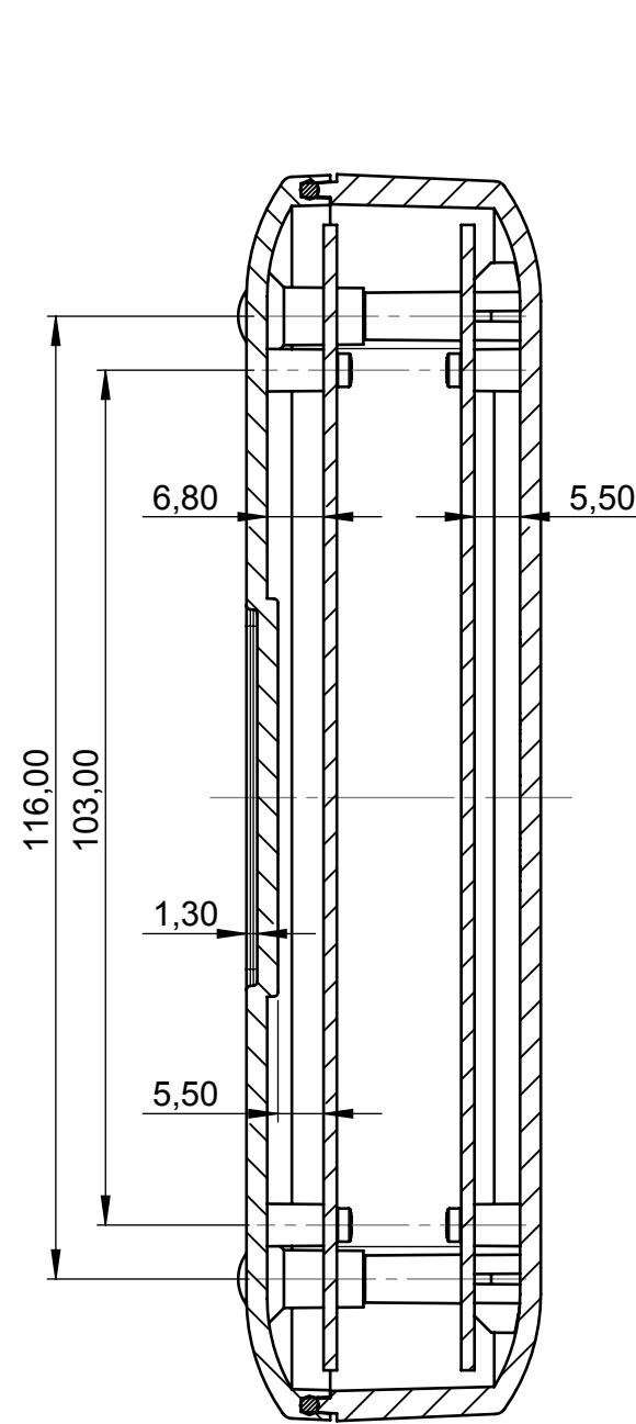
Schnitt B-B Section B-B
